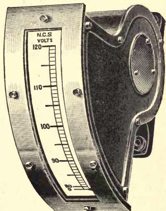
Fig. 34.—"N.C.S." Edgewise Voltmeter
